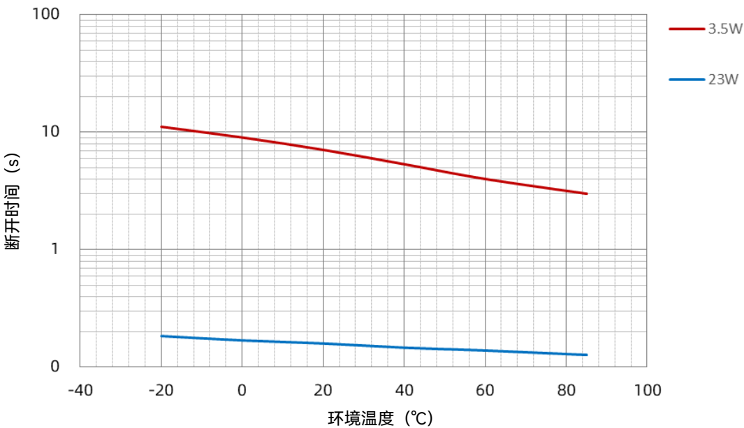
SHG 12 A 功率-温度曲线
