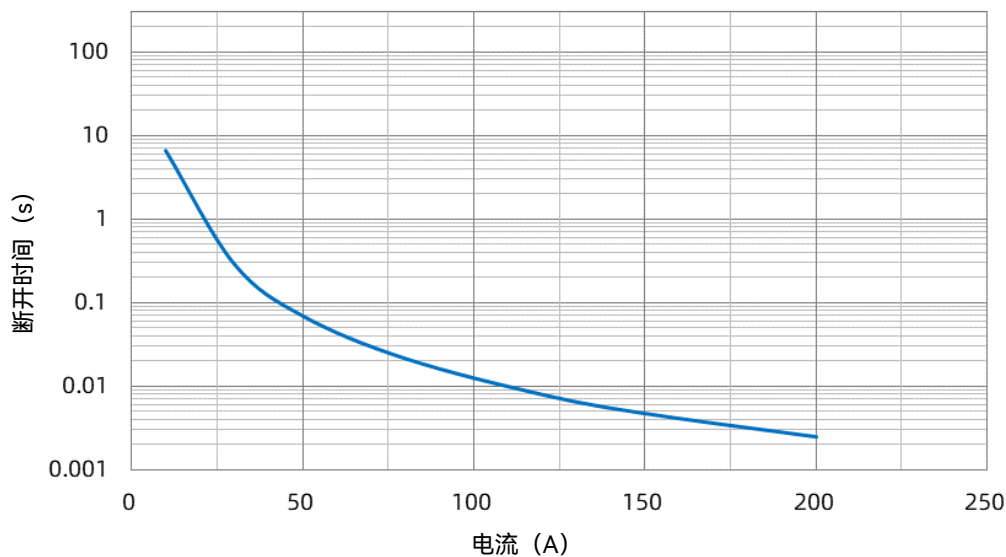
SHG 12 A 电流-时间曲线
