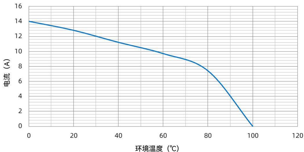
SHG 12 A 载流能力曲线
