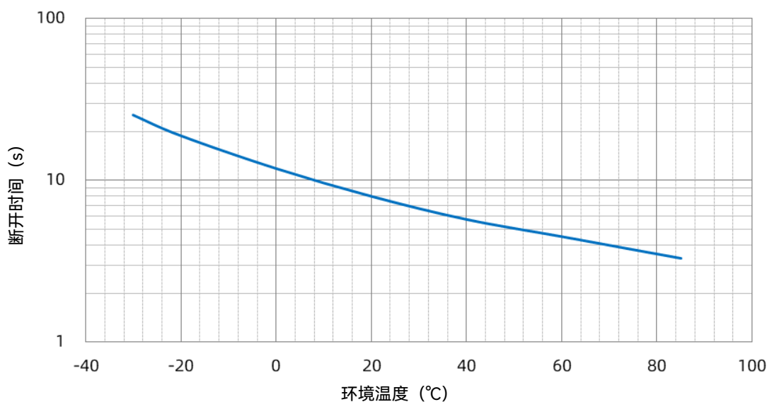
SHG 12 A 温度-时间曲线
