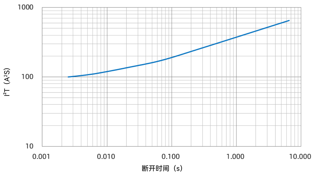
SHG 12 A I 2 t-t 曲线
