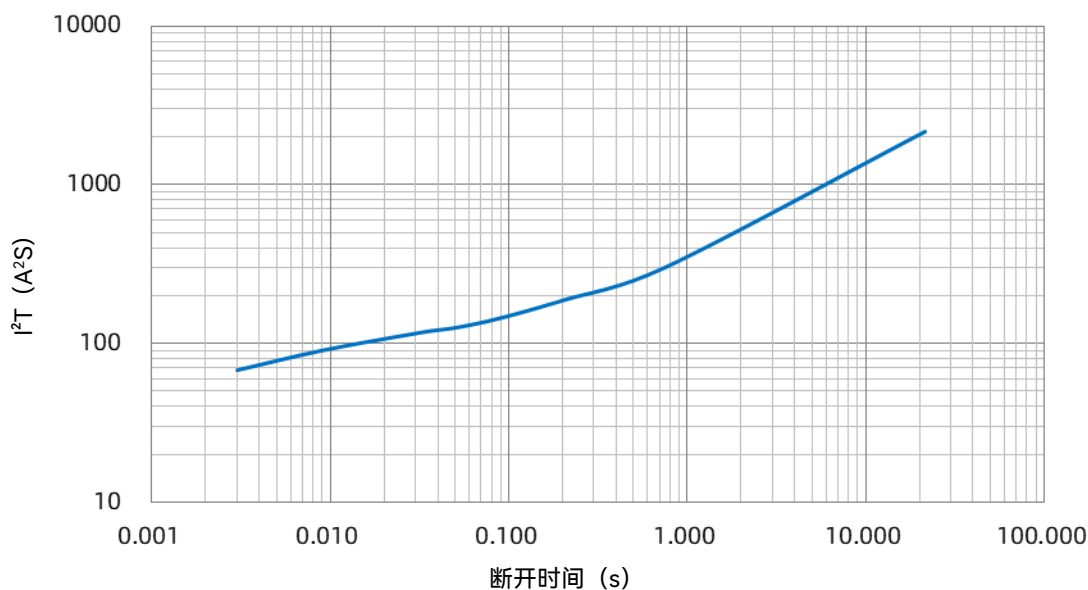
SHG 05 A I 2 t-t 曲线
