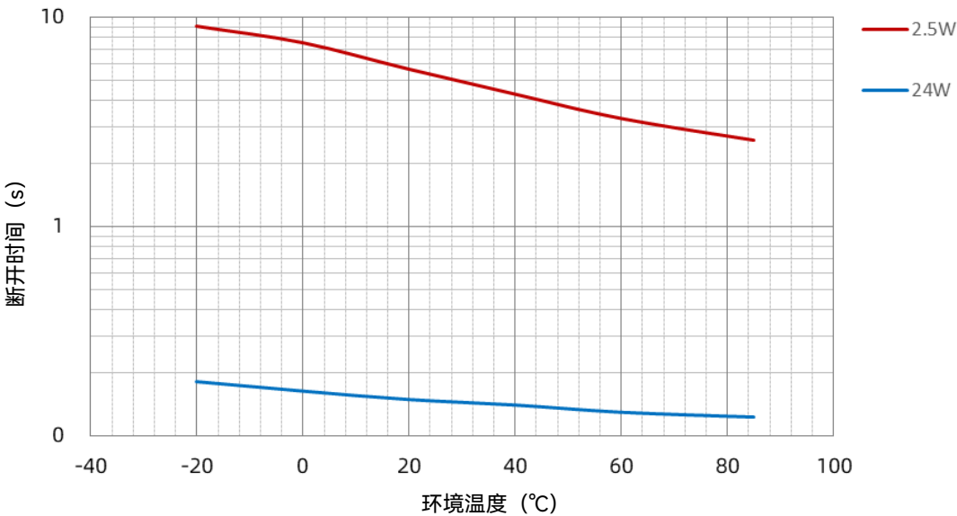
SHG 05 A 功率-温度曲线
