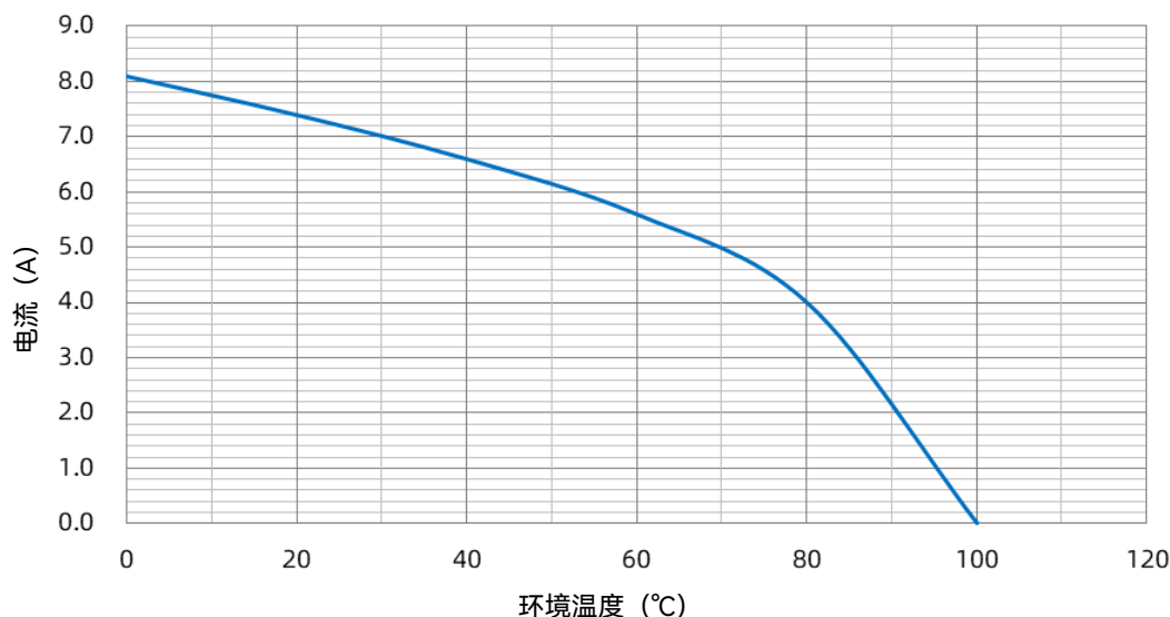
SHG 05 A 载流能力曲线
