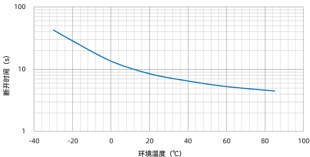
SHG 05 A 温度-时间曲线
