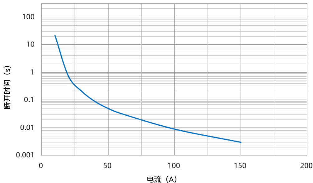
SHG 05 A 电流-时间曲线
